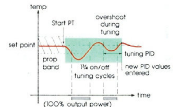
Fig. 2 Autotune PT
