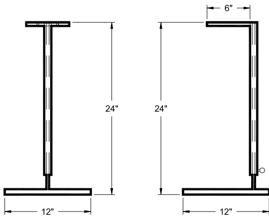
RING STAND
